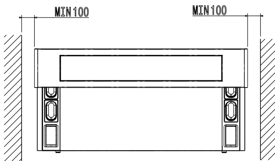
Felülnézet
